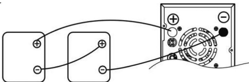
Рисунок 1. Пример подключения модели 1000 Online
